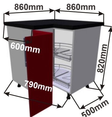
Spodní roh ODP levá LESK ROH ODP 690/3-4 L 86x82x86
